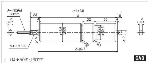
寸法図 φ48.6/φ50
