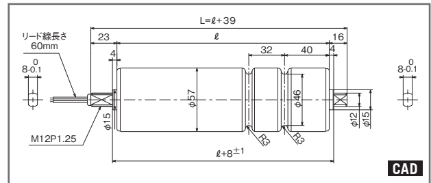
寸法図 φ57
