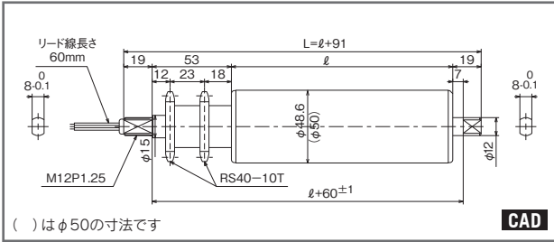
寸法図 φ48.6/φ50
