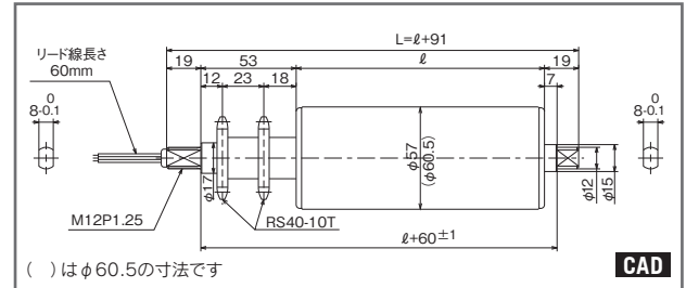
寸法図 φ57/φ60.5
